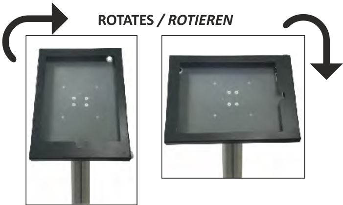
Rotation of Fixing Brackets Die Drehung der Befestigungswinkel
